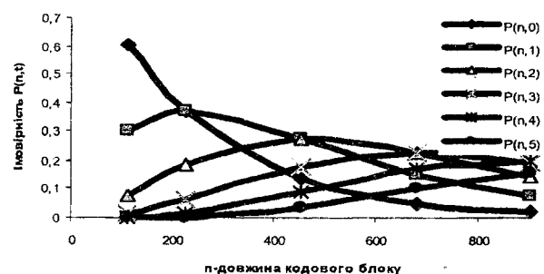
Рис. 3. Залежність статистичної P(n,0) та P(n,t) від довжини кодового блоку для КХ ВП
