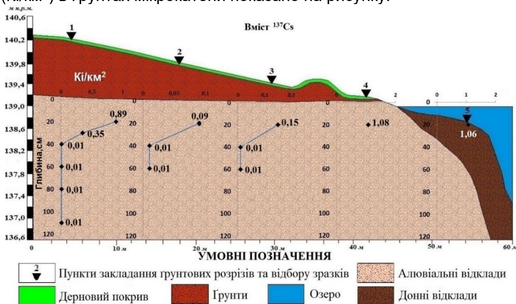
Рис.1. Модель ґрунтово-геохімічної мікрокатени водозбору оз. Миляцьке, яка відображає радіальний розподіл ^{137}\text{Cs}
