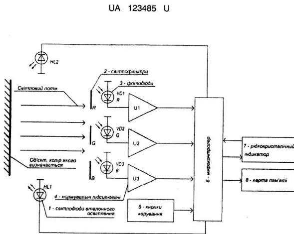
Рис. 1 – Цифровое портативное устройство измерения цвета
